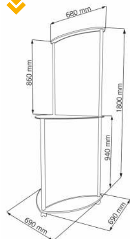
Wymiary trybunki
