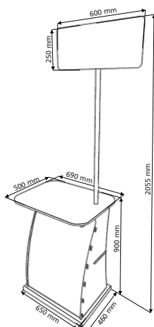
Wymiary stoiska
