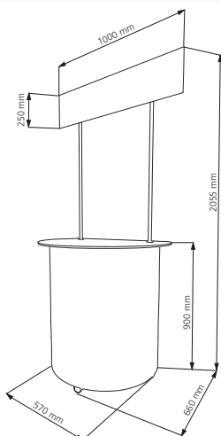
Wymiary stoiska
