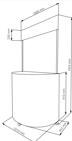
Wymiary stoiska
