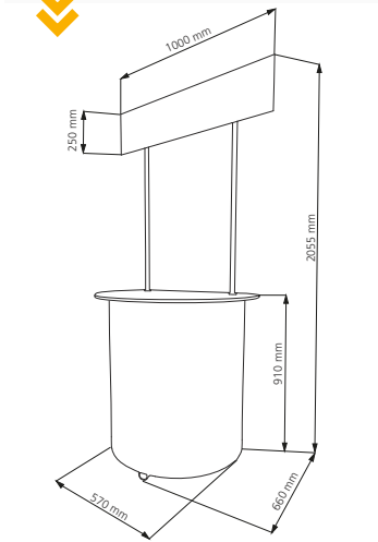
Wymiary stoiska
