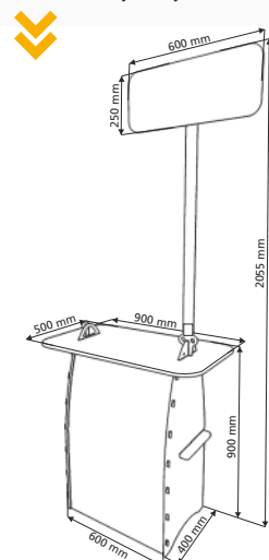
Wymiary stoiska
