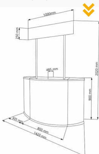
Wymiary stoiska
