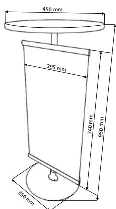
Wymiary stoiska
