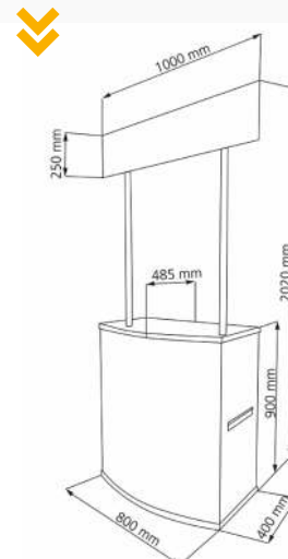
Wymiary stoiska
