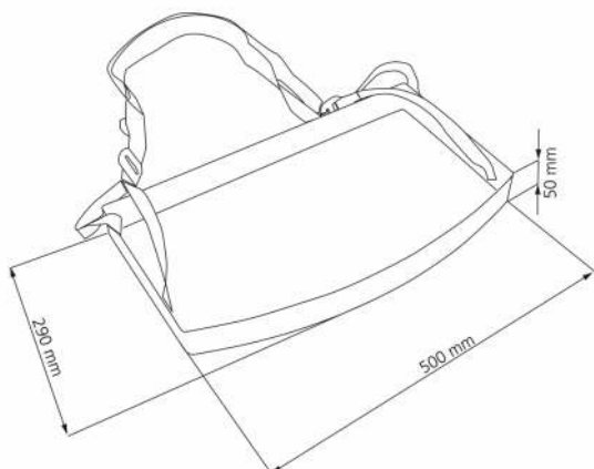
Wymiary tacki
