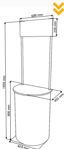
Wymiary stoiska
