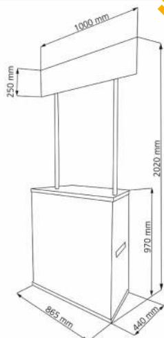
Wymiary stoiska
