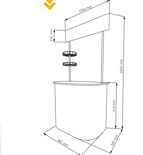
Wymiary stoiska
